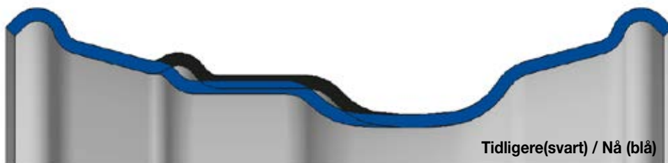
Felg med sikkerhetshump
